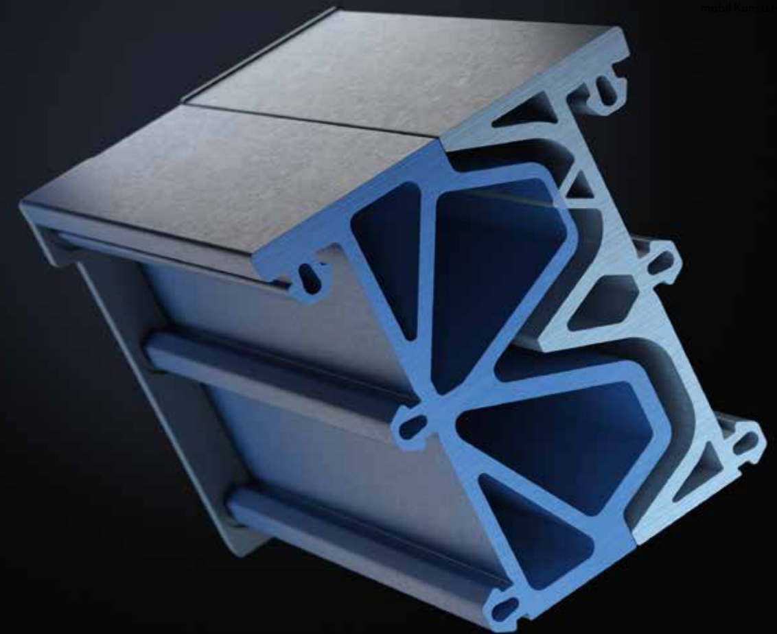
Nachbearbeitete Profile
